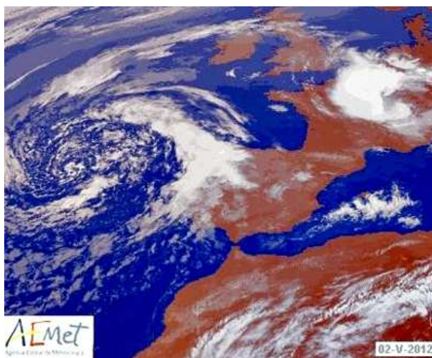
9.-Imagen infrarroja Meteosat (26-IV-2012)
