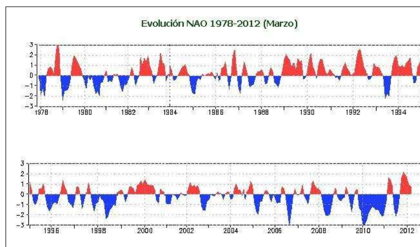
Gráfico 6: Evolución de los índices de la NAO por años y meses
