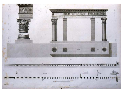
Figura 1. Elementos del templo de Marte empleados en la remodelación del hornito de Santa Eulalia. Según A. Laborde.
