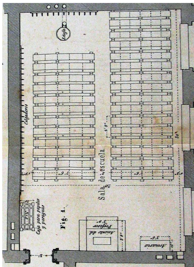
Modelo de Escuela creado por JAREÑO Y ALARCÓN, F. en 1870. En: Memoria facultativa sobre los Proyectos de escuelas de Instrucción Primaria (premiados en concurso público, adquiridos por el Estado y mandados publicar por Decreto de S. A. el Regente del Reino de 7 de abril de 1870). Madrid, Imprenta Nacional de Sordo-Mudos y de Ciegos. 1871.
